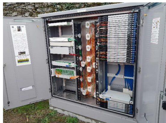
Armoire après le raccordement final de plusieurs locaux
